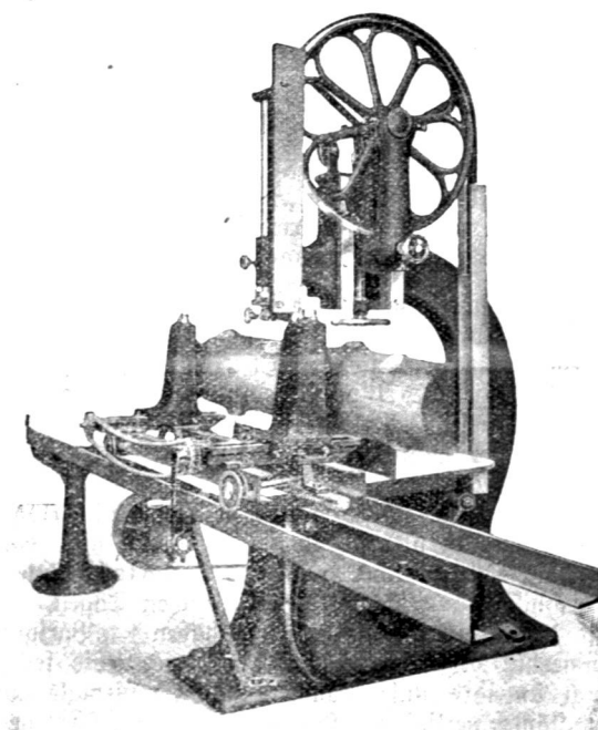
Bandsäge mit Laufwagen mit selbsttätigem Vorschub.
