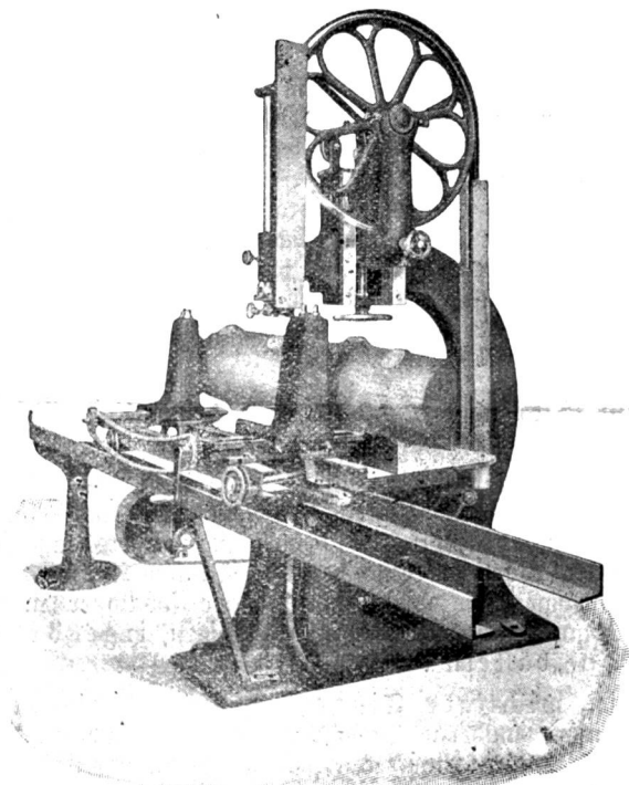
Bandsäge mit Laufwagen mit selbsttätigem Vorschub.
