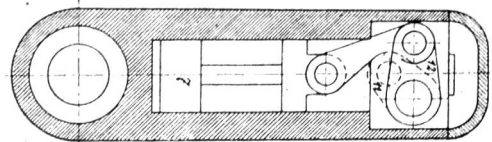
Fig. 2 Draufsicht
