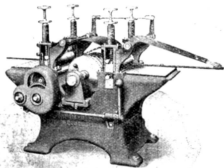
Latten-Kreissäge.
