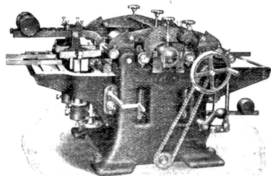
Dreseitige Hobelmaschine.
