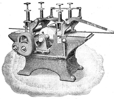
Latten-Kreissäge
