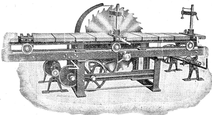
Kantholz- und Besäum-Kreissäge.
