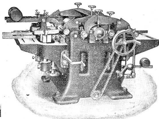
Dreseitige Hobelmaschine.
