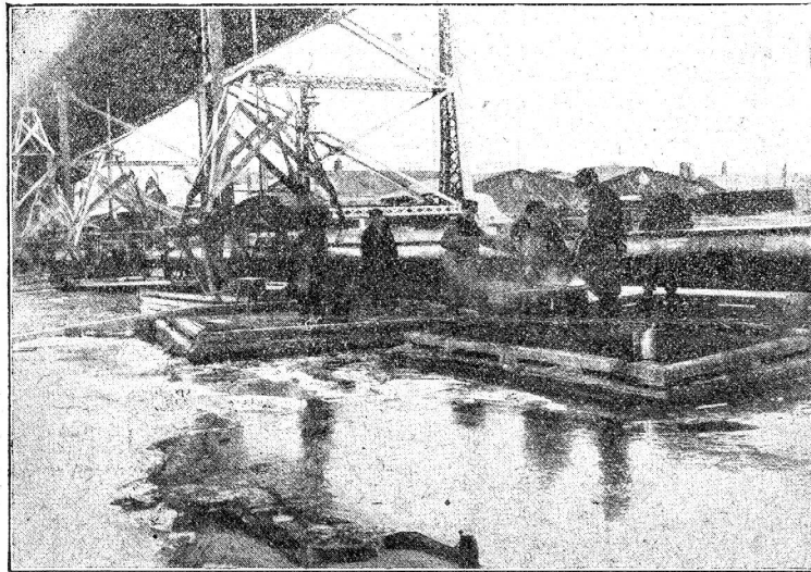
Verlegung eines Dückers aus Flanschenröhren von 600 mm I. W., in Klaraviken, Wasserleitung STOCKHOLM.
