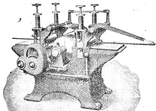
Latten-Kreissäge
