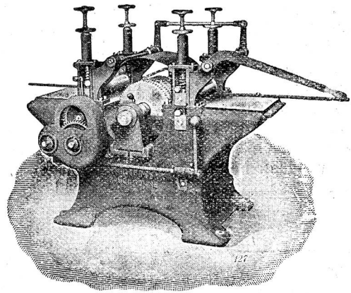
Latten-Kreissäge
