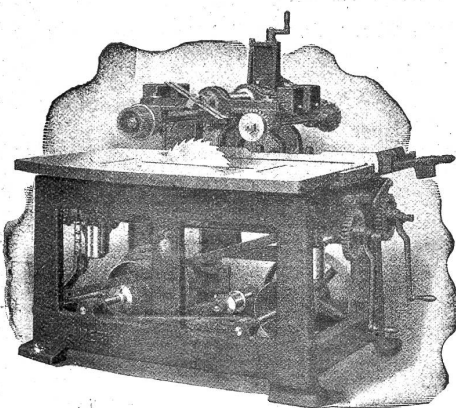
Kreissäge mit mechanischem Vorschub
