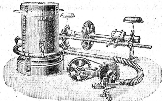
Abbildung 10. Gas-Schmelzgebläse.
