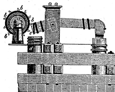
Abb. 8. Mechanischer Stielhammer, mit Wasserkraft betrieben.
