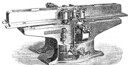
Nut-, Spund- und Fügemaschine für konische und parallele Bretter
