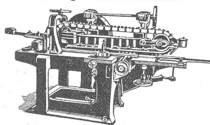
Vierseitige Parkethobelmaschine
