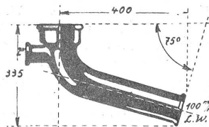
Fig. 1006 Klosettbogen mit 2" Gewindeanschluß für Bad oder Wandbecken
