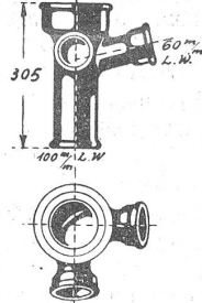
Fig. 1003 mit zwei 75 gradigen Muffen- anschlüssen von 60 mm Lichtweite
