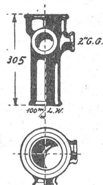
Fig. 1001 mit zwei 2" Gewindeanschlüssen
