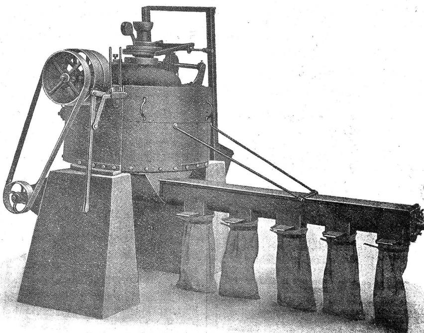
Abb. 6. Staubbicht abgeschlossene Trockenmischmaschine „Pat. Strich“ mit automatischem Rohmaterialaufzug, Transportschnecke und Absackvorrichtung
