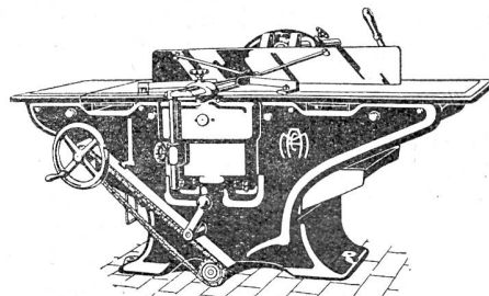
Kombinierte Abricht-, Kehl- und Dickenhobelmaschine 36h Mod. H. D. — 360, 450, 530 und 610 mm Hobelbreite
