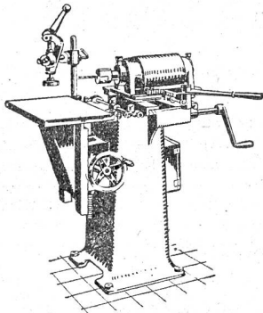
LBM: Riemenlose Langloch-bohrmaschine mit eingebautem Elektromotor.
