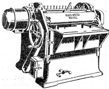
Riemenlose Gliederwalzen- Dickenhobelmaschine.
