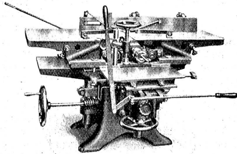
UNIVERSAL - KOMBINIERTE HOBELMASCHINE H. E. K. mit Kreissäge und Bohrmaschine 13
