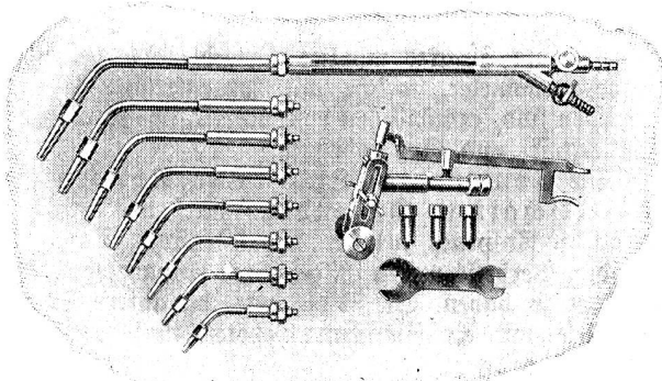
Schweiß- und Schneidbrenner „Progreß“ mit auswechselbaren, flammenrückschlagssicheren Einfäßen.
