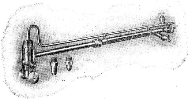
Brauguss-Schneidbrenner „Continental“.
