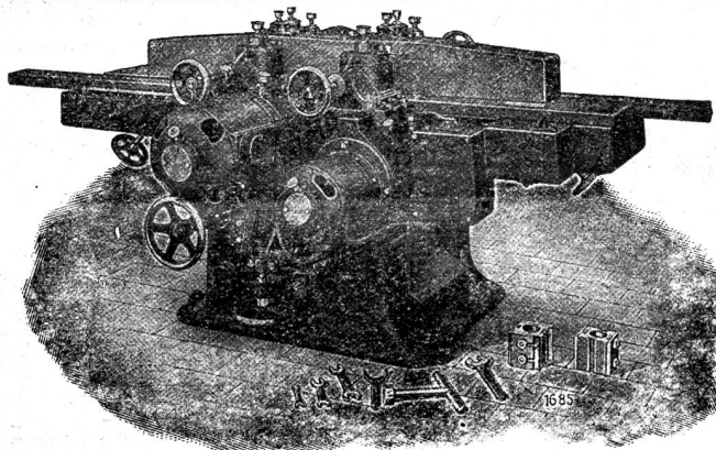
DSPM Automatische doppelseitige Nut und Spundmaschine
