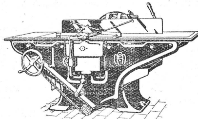
Kombinierte Abricht-, Kehl- und Dickenhobelmachine 2 b Mod. H. D. — 360, 450, 530 und 610 mm Hobelbreite
