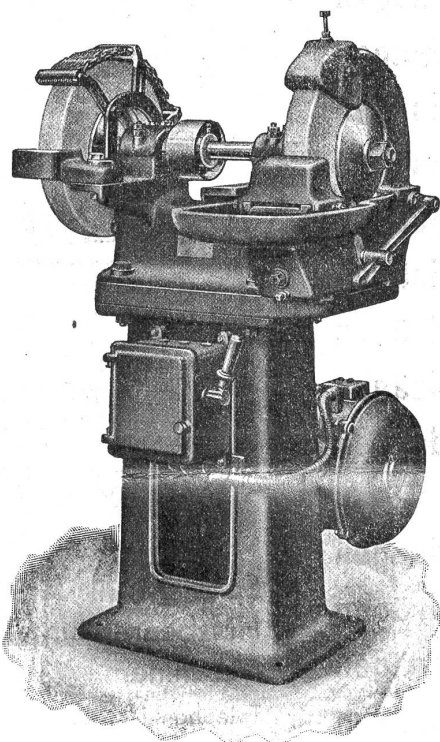
Mod. 30 b mit Einzelantrieb für Scheiben von 350x60 mm
