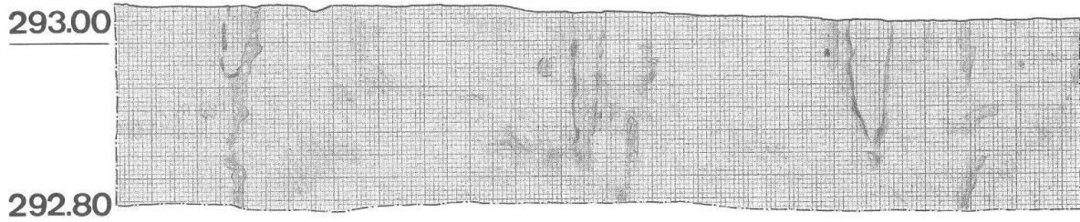
Abb. 18 Augst, Insula 22 (Grabung 1988.51): Drei geschnittene Pföstchen P116, später teilweise durch Wurzelgänge erweitert. M. 1:30.
