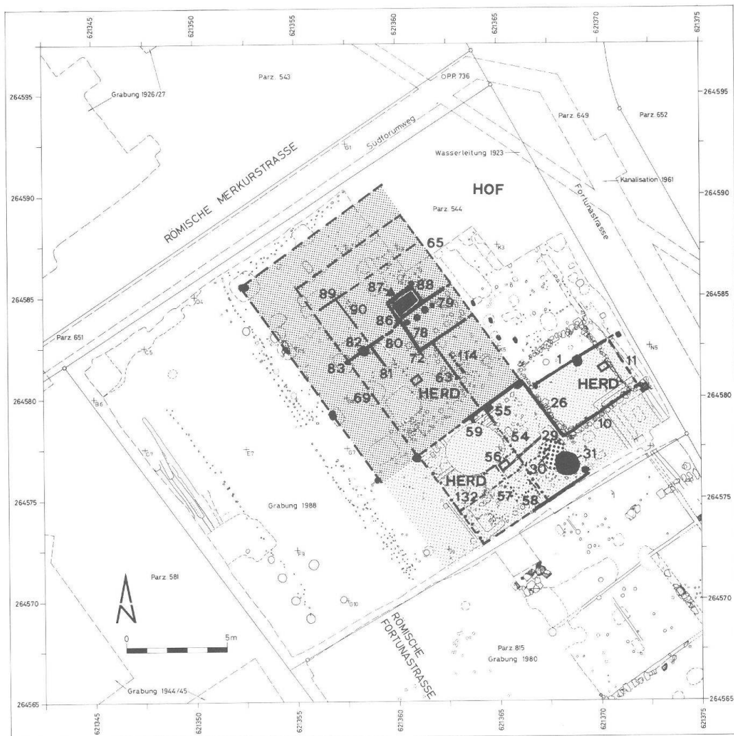
Abb. 25 Augst, Insula 22 (Grabung 1988.51), Bauzustand 3. M. 1:250.
