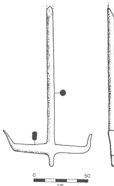
Abb. 8: Spätromischer Anker mit abgeknickten Armen aus Dor/Tantura, Israel. M. 1 : 20.
