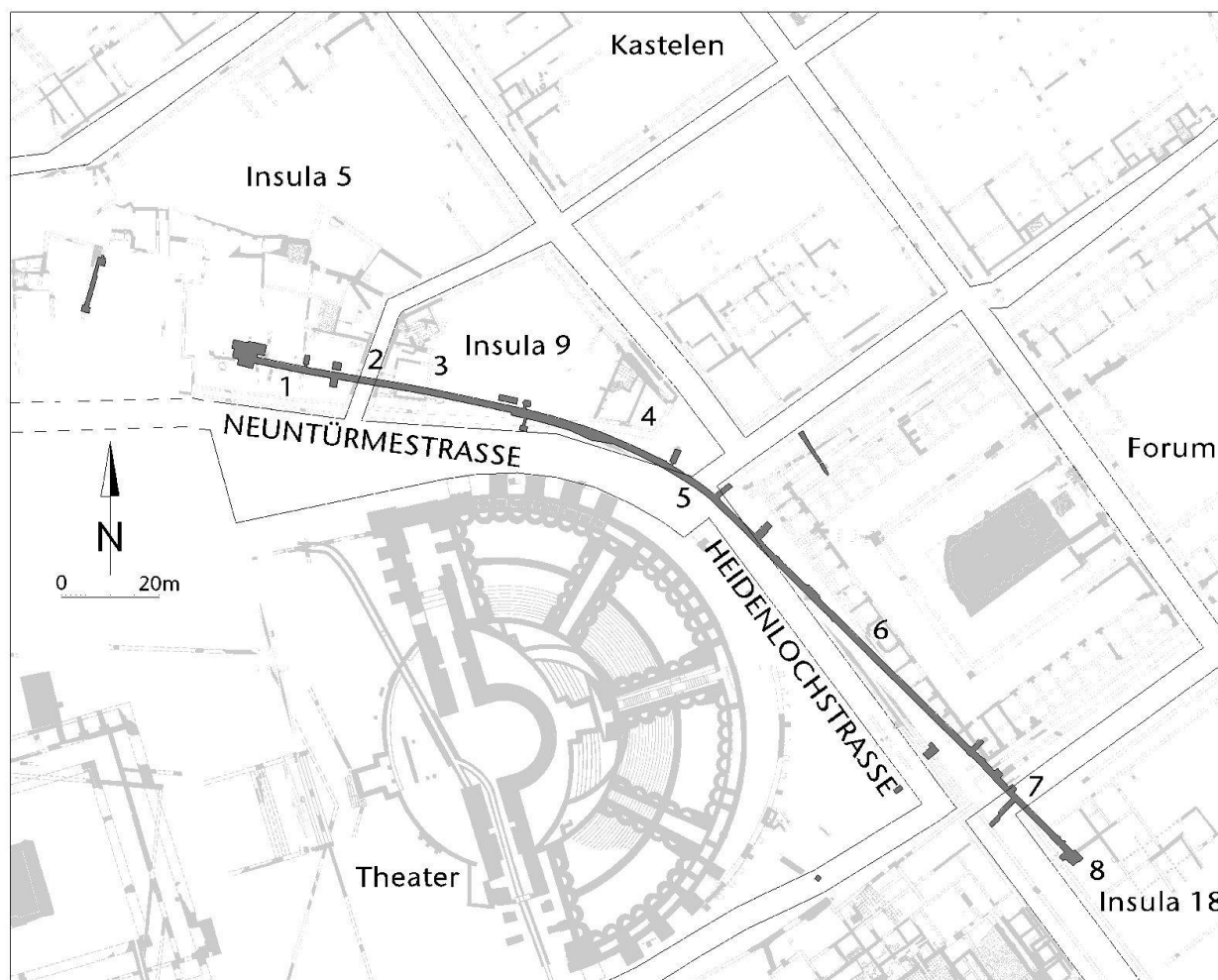
Abb. 2: Augst BL, Wasserleitung Giebenacherstrasse (Grabung 2003.51). Der Verlauf des Grabens im römischen Stadtgebiet. Eingezeichnet sind die Sektorenummern 1–8, nach denen die Befunde im Text beschrieben sind. M 1:1500.
