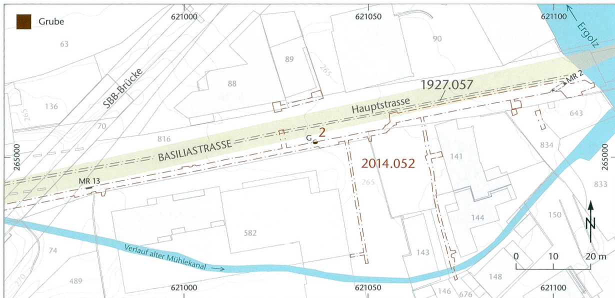
Abb. 15: Augst BL, Wasserleitung Hauptstrasse (Grabung 2014.052). Abschnitt des Leitungsgrabens zwischen Ergolzbrücke und SBB-Brücke mit Eintrag der römischen Grube G (vgl. Abb. 10,2). Die eingetragene Mauer MR 2 ist nachrömisch. M. 1:1 000.
