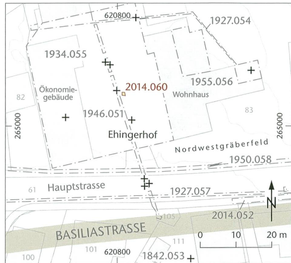
Abb. 60: Augst BL, Vorplatz Ehingerhof (Grabung 2014.060). Situationsplan mit dem Leitungsgraben von 1946 und den dabei gefundenen Brandgräbern (Kreuze). M. 1:1 000.
