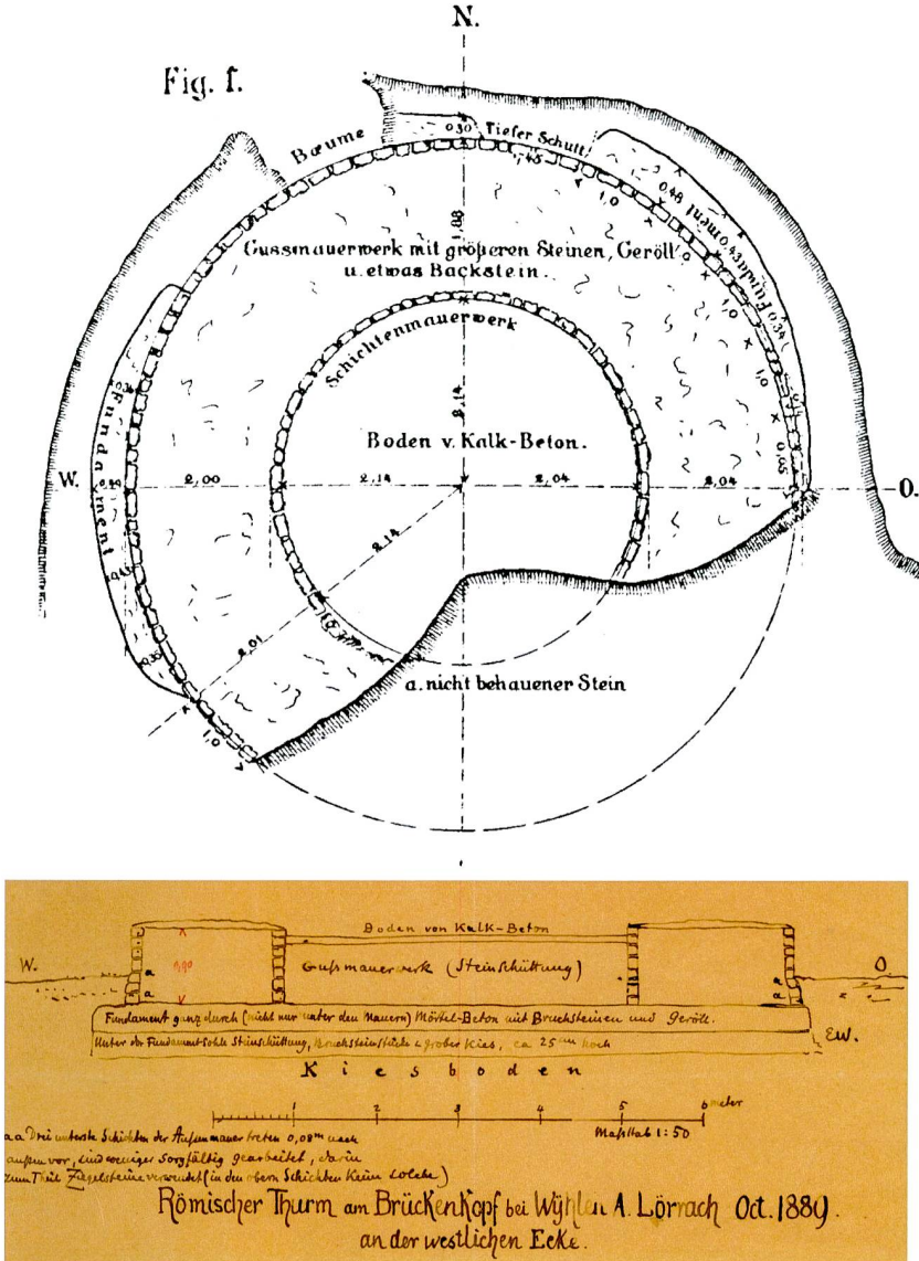
Abb. 4: Wyhlen (D), Brückenkopf. Grabungen E. Wagner 1887/1889. Oben: Grundriss Turm I. Unten: Querschnitt Turm I. M. 1:100.
