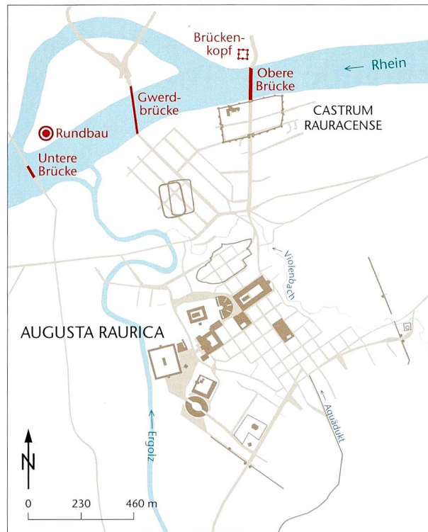
Abb. 1: Übersichtsplan von Augusta Raurica (Augst BL und Kaiseraugst AG). Situation der drei Rheinbrücken in der heute üblichen Darstellung. M. 1:23 000.
