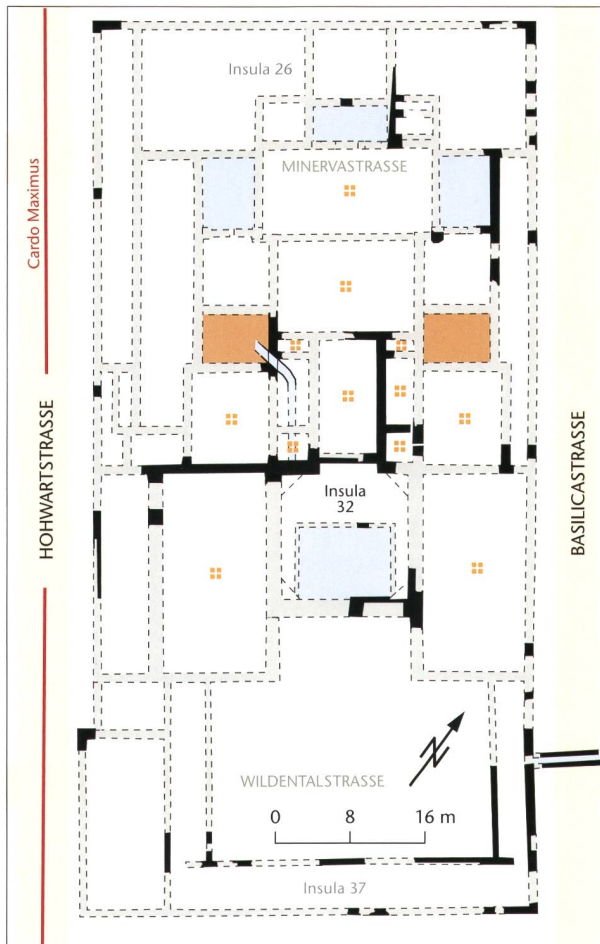
Abb. 32: Augusta Raurica. Vereinfachter Übersichtsplan der Zentralthermen zwischen der Basilica- und der Hohlwartstrasse (Cardo Maximus). Gut zu erkennen sind die beiden im Zuge einer Thermenerweiterung überbauten West-Ost verlaufenden Strassenzüge der Minerva- und der Wildentalstrasse. M. 1:800.
