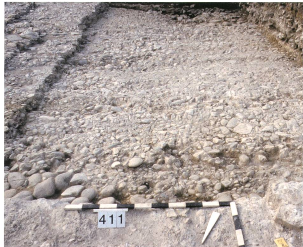
Abb. 2: Augusta Raurica. Karrenspuren in einem Kieskoffer der West-Ost verlaufenden Silberschatzgasse (Grabung 1997.004). Blick von Norden.
