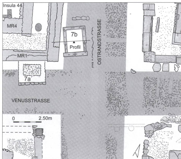
Abb. 23: Augusta Raurica. Kreuzung Venus-/Ostrandstrasse. Lage der beiden Laufbrunnen 7a und 7b (Grabung 1971.053, vgl. Abb. 25,7a.7b). Bezeichnungen der Laufbrunnen nach Furger 1997. M. 1:200.
