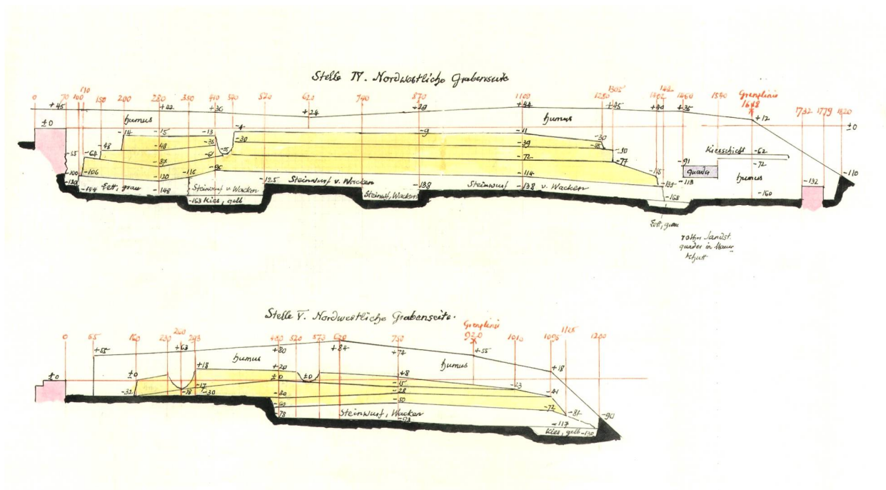
Abb. 15: Augst BL, Obermühle (Grabung 1930.055). Ansicht von Südosten an die beiden Profile durch die Raurekastrasse. Der im Text erwähnte Graben im Strassenkoffer ist in der linken Strassenhälfte («Stelle IV», Profil oben) bzw. in der Mitte («Stelle V», Profil unten) zu erkennen. Zur Lage der Profile vgl. Abb. 10. Ohne Massstab.
