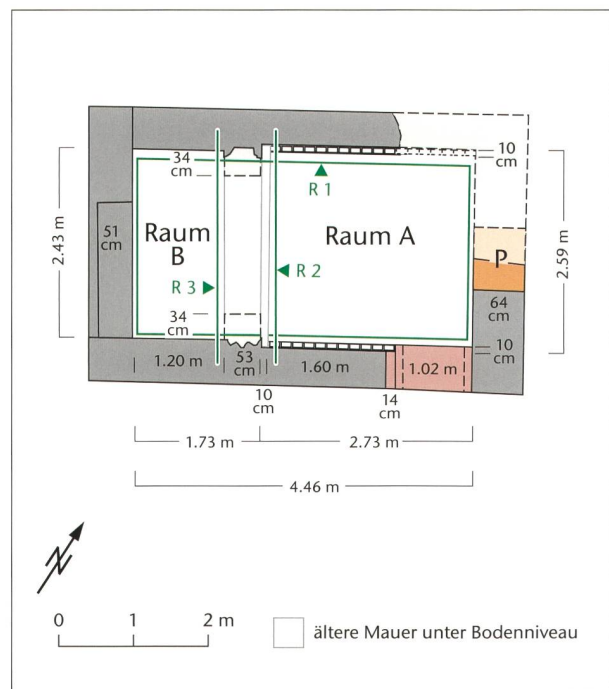
Abb. 6: Augst BL, Insula 8 (Grabung 1918–1919.051). Detail der Räume A und B mit den genauen Massen. R1–R3 = Rekonstruktionen 1–3, siehe Abb. 62. M. 1:100.
