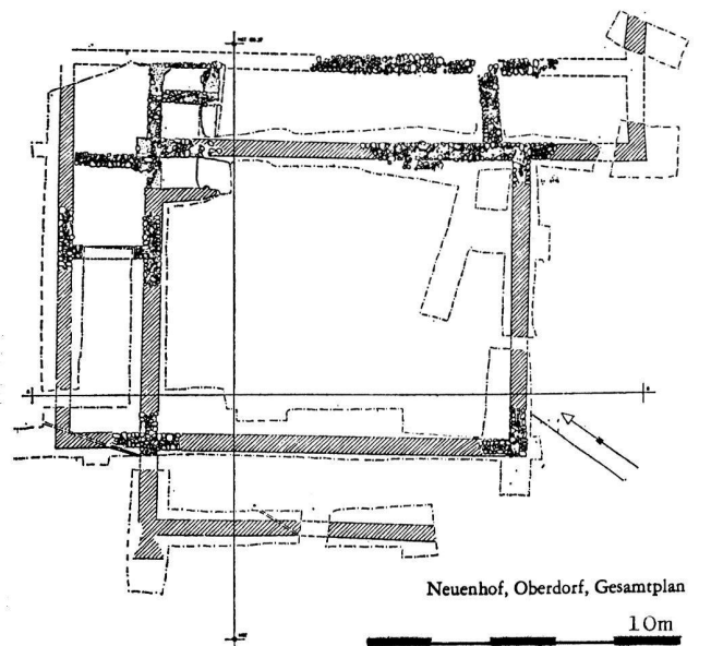
Abb. 22. Neuenhof AG, Oberdorf. Fundamente eines römischen Gebäudes mit offenem Innenhof. Katasterplan (oben) und Grundrissplan (unten).
