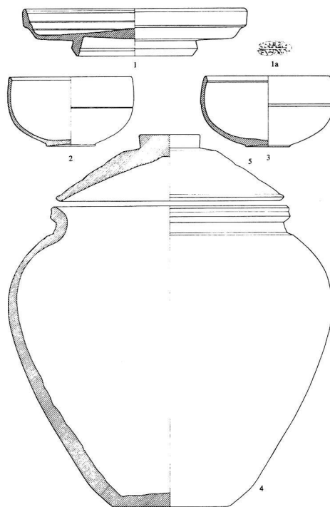
Abb. 36. Windisch AG, Vindonissa, Alte Zürcherstrasse, 1973. Urne und Beigaben aus dem Ziegelkistengrab. Gefässe M. 1 : 4, Stempel M 1 : 2. (Zeichnung R. Baur).
