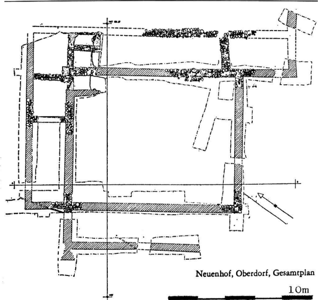
Abb. 22. Neuenhof AG, Oberdorf. Fundamente eines r mischen Gebudes mit offenem Innenhof. Katasterplan (oben) und Grundrissplan (unten).
