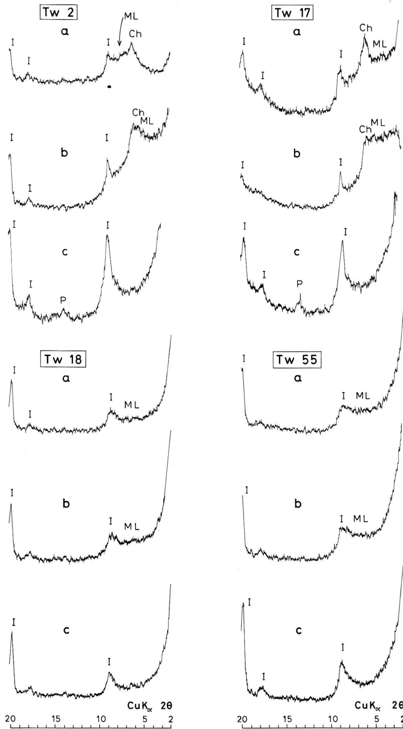
Abb. 10: Ausgewählte Texturpräparate der vier Scherbengruppen aus Twann, a = normales, lufttrockenes Präparat, b = glykoliertes Präparat ( 60^\circ\text{C}/24\text{h} ), c = gebranntes Präparat ( 550^\circ\text{C}/1\text{h} ). Ch = Chlorit, I = Illit, ML = Mixed-layer, P = Plagioklas.
