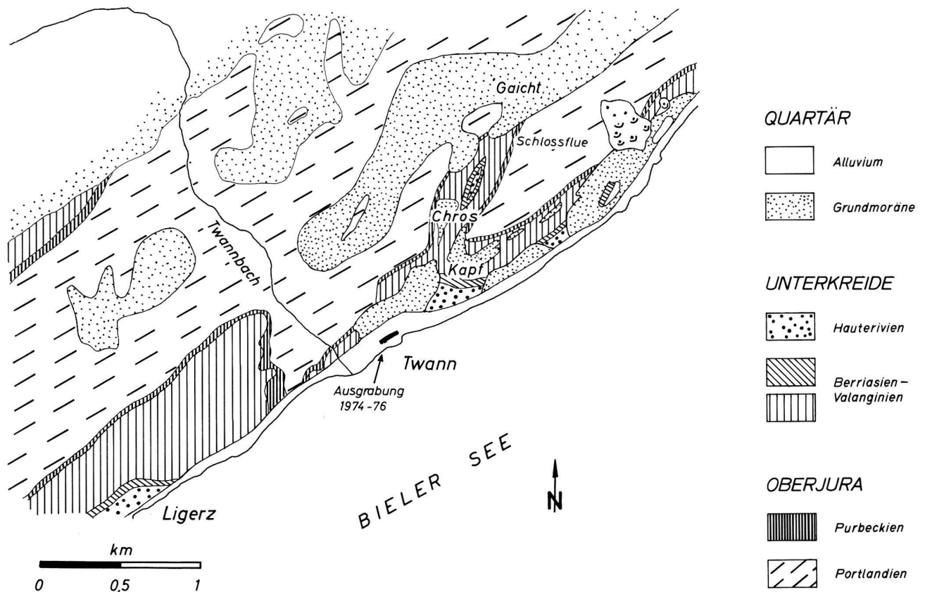
Abb. 13: Geologische Situation von Twann und Umgebung, vereinfachte Karte nach Geol. Atlas der Schweiz, 1:25 000, Blatt 1145 «Bieler See». Signaturen für Berriasien-Valanginien: Marnes d'Arzier, Calcaire roux Mergel- und Kalkzone, Marbre bâlard Das Rohmaterial der Keramik entstammt demjenigen Gelände um Twann, das, damals bis heute, kultiviert worden ist: dem Bereich der Grundmoräne und der Unterkreide-Mergel.
