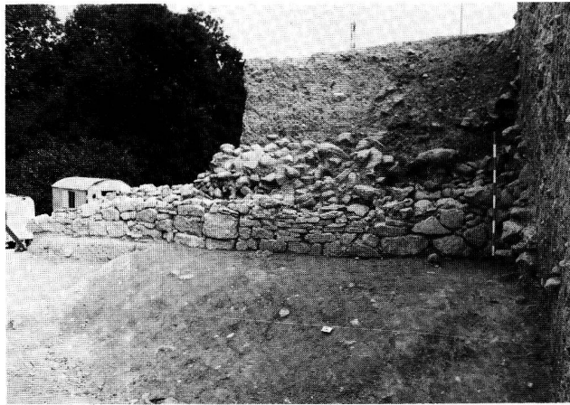
Fig. 27. Gressy VD, Butte de Sermuz. Murus gallicus, parement interne. Photo P. Curdy.
