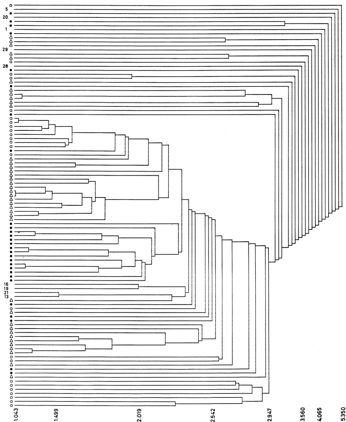
Abb. 15. Clusteranalyse der drei Augster Referenzgruppen und der Amphoren. Auf der Ordinate sind eingetragen: Nr. (Amphoren), Kreise (Kurzenbetti CA), Dreiecke (Osttor), Punkte (Venusstrasse CA). Auf der Abszisse sind ausgewählte Verknüpfungs- bzw. Amalgamationswerte angegeben. Die Abbildung zeigt die Streuung bzw. Vermischung der drei Referenzgruppen, aber auch die niedrigen Verknüpfungswerte für die Mehrzahl der Proben. Ein Teil der Amphoren gruppiert sich (4 Analysen), eine anderer Teil ist randlich gestreut (5 Analysen).
