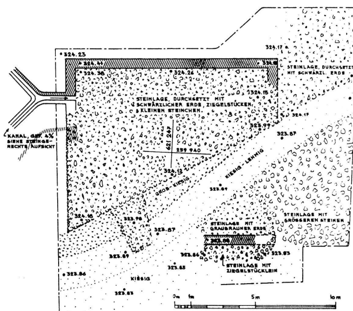
Abb. 32. Liestal BL, Munzach. Gutshof, Nebengebäude 15 (Grabung Brühl 1968). Nach Dokumentation AMABL.
