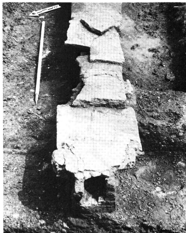
Fig. 10. Orbe VD, Boscéaz. Trois exemples de canalisations découvertes en 1987: a) conduit de maçonnerie couvert par des tegulae et des imbrices (flèche), se jetant dans le collecteur principal voûté. b) canal formé d'éléments de terre cuite en U, emboîtés et couverts de tegulae retournées. c) vue à l'intérieur du collecteur principal.
