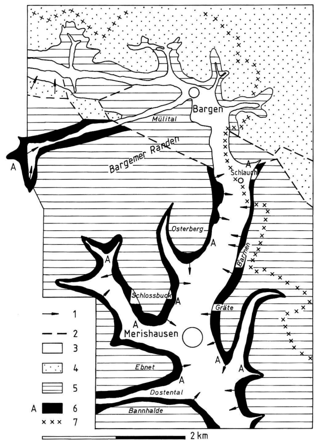
Abb. 5. Geologische Übersichtskarte des nördlichen Durachtales zwischen Merishausen und Barmen. 1 Rutschungen (Gehängeschutt, Schuttkegel). 2 Geologische Störung (Randenerverwerfung). 3 Talfüllung (Alluvionen). 4 Tertiäre Ablagerungen. 5 Malm. 6 Ausstrichflächen der Schichten im Übergangsbereich Dogger/Malm (oberes Callovian, tieferes Oxfordian); A = Aufschlüsse in den Macrocephalus-Schichten. 7 Landesgrenze.
