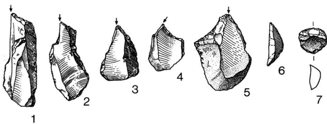
Abb. 1. Egolzwil LU, Gere. 1–5 Stichel an Endretouche (1–3 an Klinge; 4–5 an Abschlag); 6 Segmentmesser; 7 Mikrokratzer. M 1:2.
