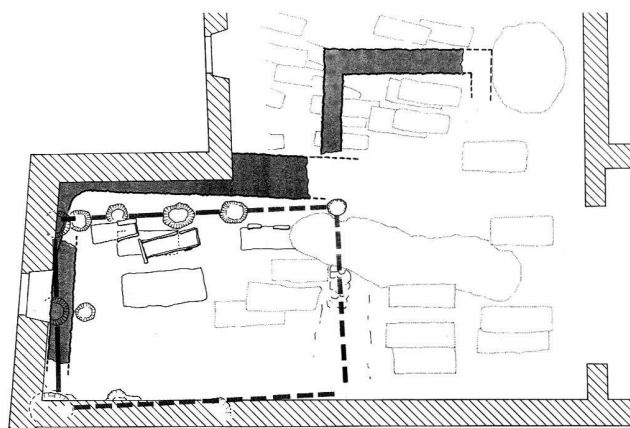
Abb. 39. Buus BL, Kirche. Westpartie der Kirche: Pfostenlöcher der Holzkirche, Gräber; punkterasterte Mauerzüge: erster Steinbau. Länge des Holzbaus: 9,4 m.
