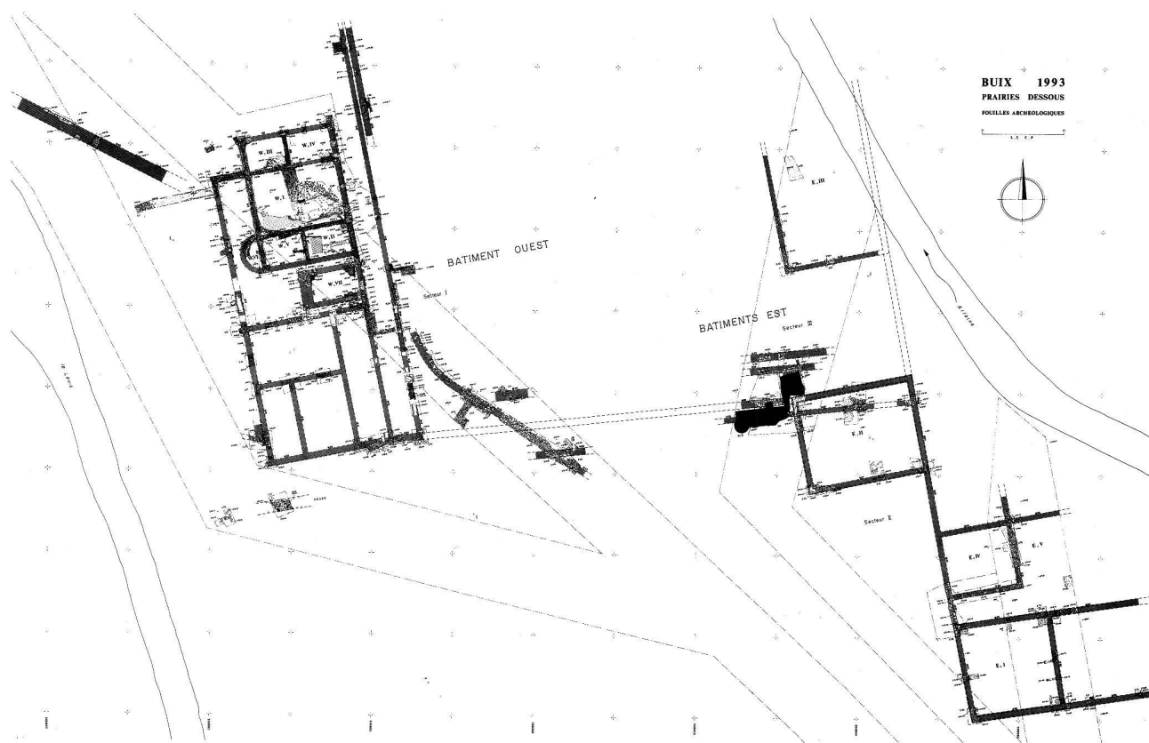
Fig. 19. Buix JU, Les Prairies Dessous. Plan général des fouilles et sondages 1993. Lignes interrompus hachurées, la restitution des murs; lignes interrompus, le trace hypothétique des murs; en grisé, les vestiges médiévaux. Ech. 1:800. Plan OPH JU.
