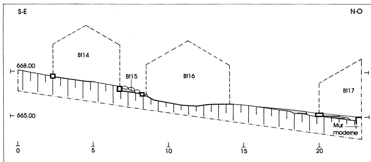
Fig. 3. Coupe schématique à travers le secteur de fouille du bâtiment 16, vue ouest. Les bâtiments 14, 16 et 17, dont le volume a été reconstitué, sont contemporains. Des niveaux plus anciens (en grisé) ont été repérés sous le bâtiment 17 et entre les bâtiments 14 et 16 (Bt15).
