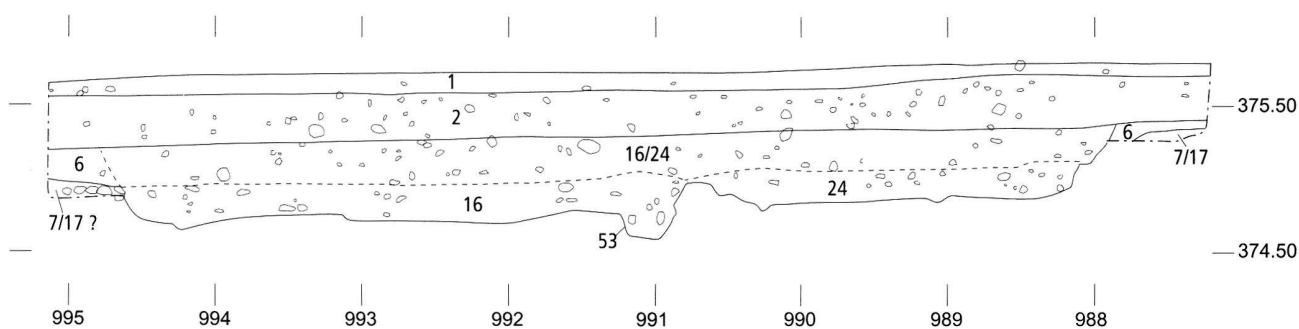
Abb. 5. Andelfingen, Flaacherstrasse 14. Profil durch die Grubenhäuser, auf Laufmeter 207,4–207,6. M 1:50. Zeichnung KA ZH, M. Moser.
