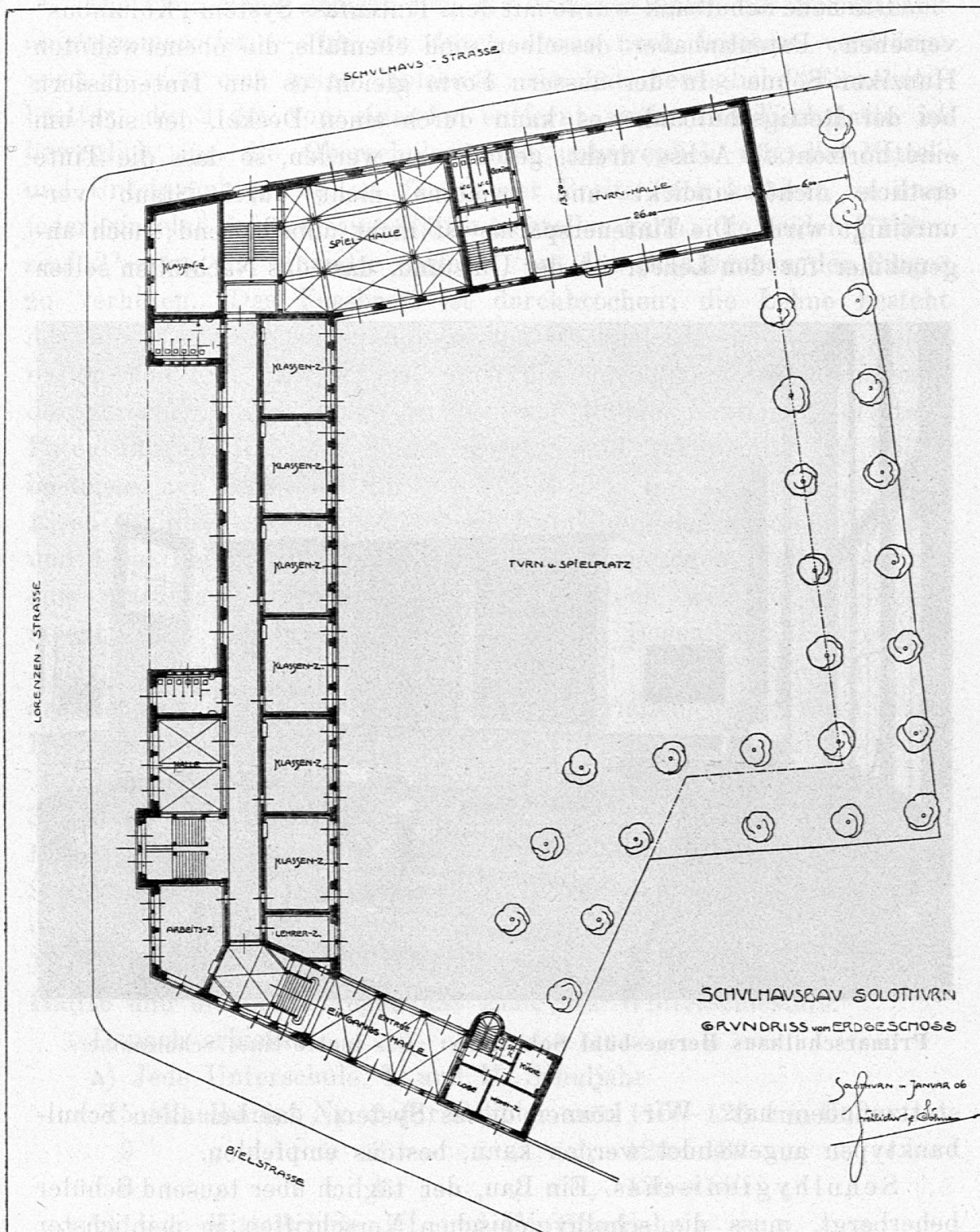
Primarschulhaus Hermesbühl Solothurn: Grundriss des Erdgeschosses.
