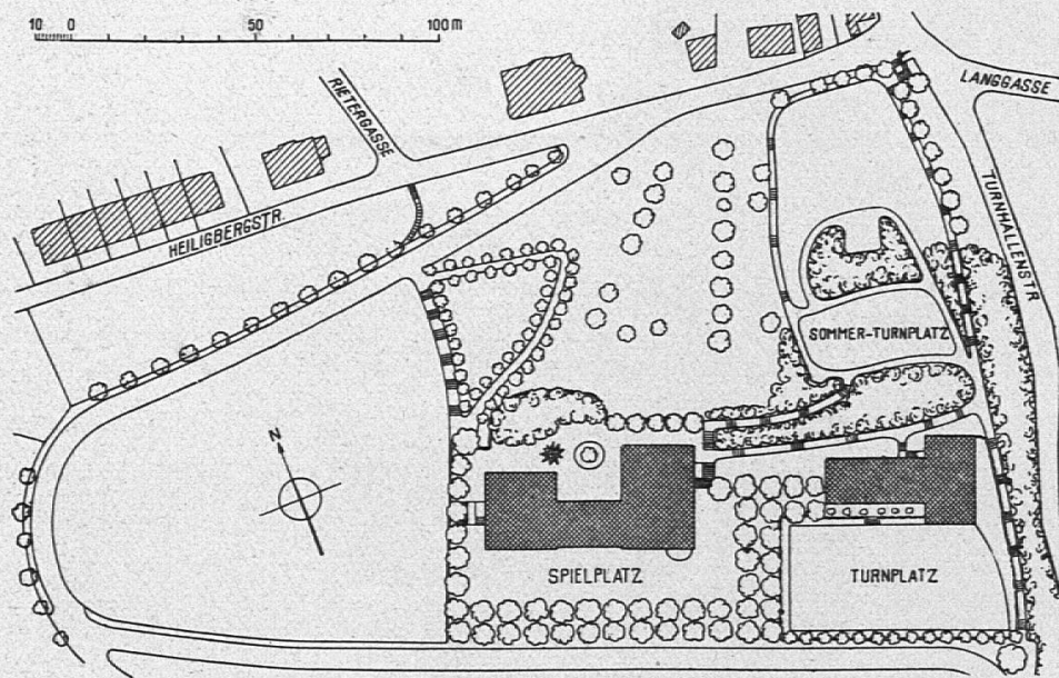
Heiligbergsschulhaus: Lageplan von Schulhaus und Turnhalle.
