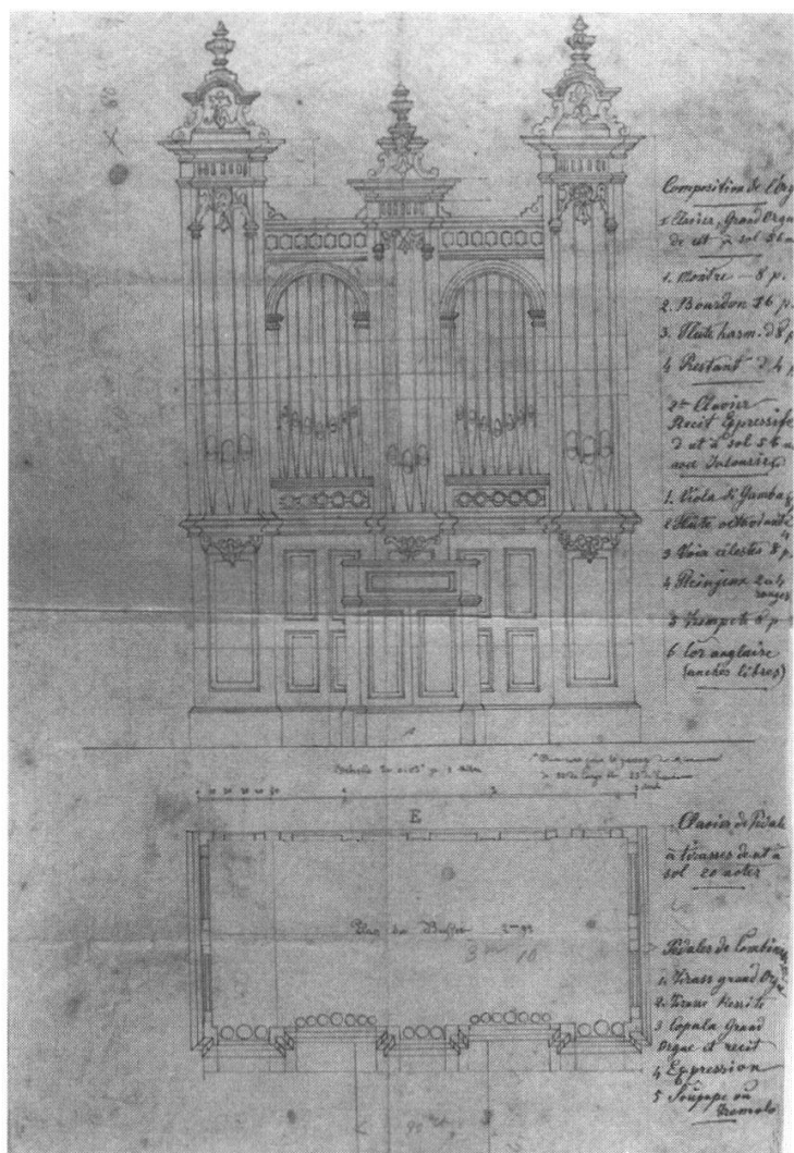
Aufriss eines Orgelprospektes in neubarockem Stil für die Franziskanerkirche von der Werkstatt Kyburz, Solothurn, um 1882 (Archiv der christkatholischen Kirchengemeinde).
