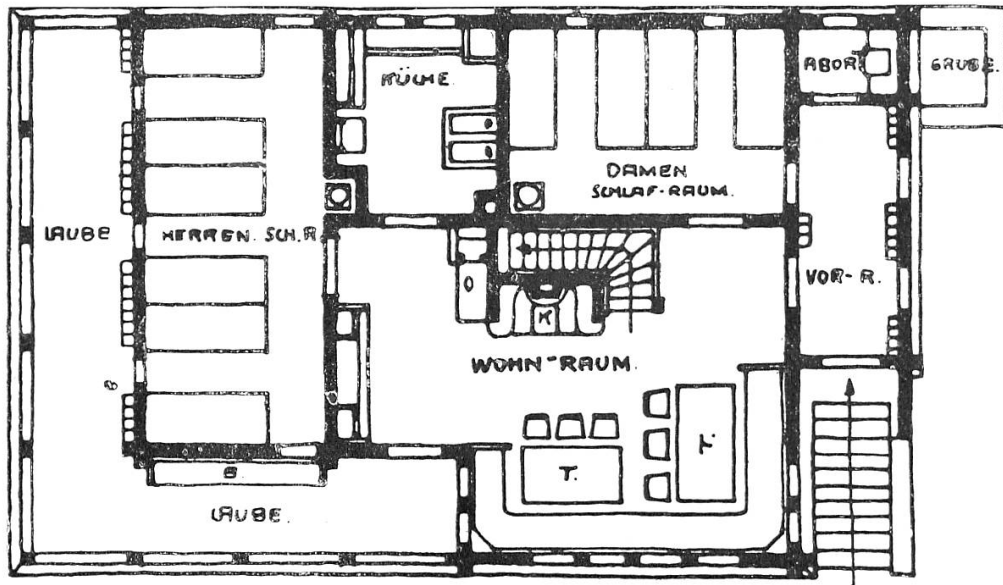
PARTERRE GRUNDRIS
