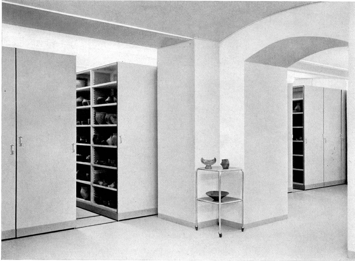
Abb. 4. Kompaktanlage aus fahrbaren und zusammenschliessbaren Schränken in der urgeschichtlichen Studiensammlung (S. 9)
