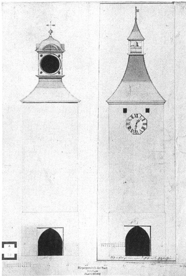
Abb. 5 Zwei Vorschläge zu einem neuen Dach auf dem Bieltor, Pläne von 1821/22. Links eine Variante, die sich den Ratshausturm von Murten zum Vorbild nahm (abgelehnt da als ungeschickt empfunden), rechts die Variante nach dem Vorbild auf dem Berntor in der Vorstadt (1825 in abgeänderter, gedrungenerer Form ausgeführt).
